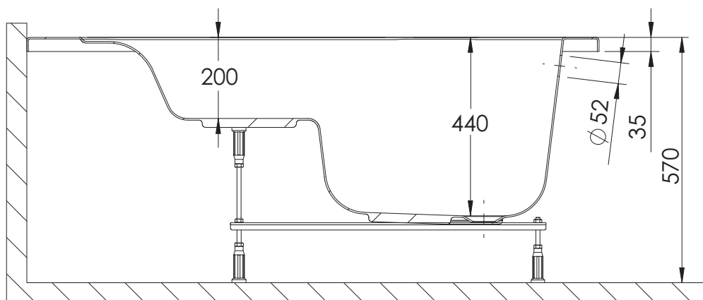
ŘEZ A-A
